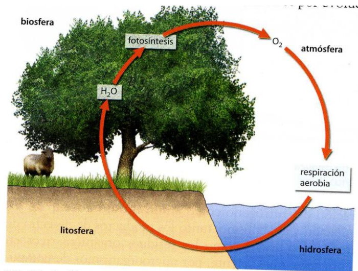
9.13. Ciclo simplificado del oxígeno.
