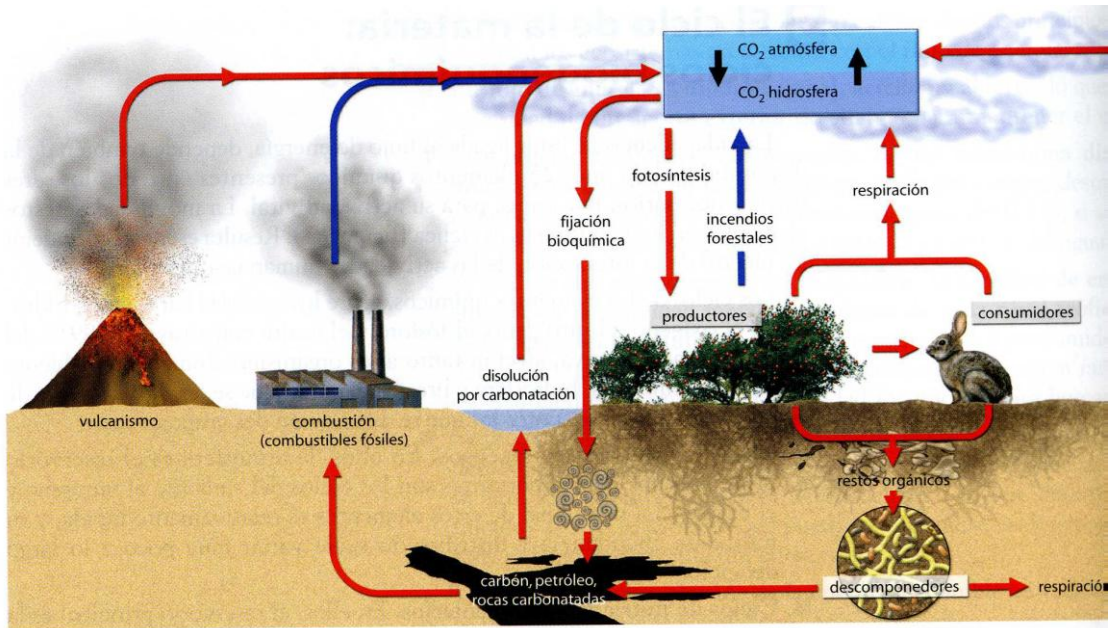
9.11. Ciclo del carbono en la biosfera.
